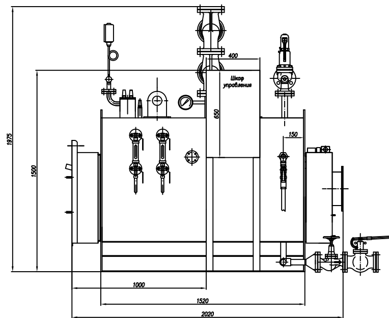
Котел 1 подключение с правой стороны
